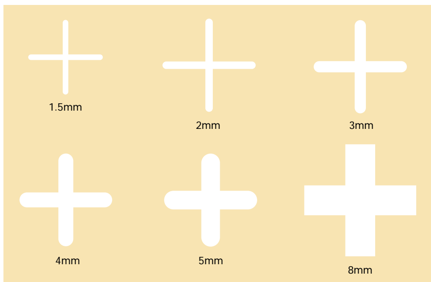
Actual size spacer profiles
